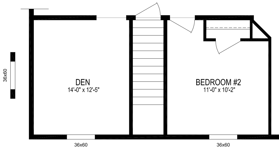
OPTIONAL BASEMENT STAIRWELL
