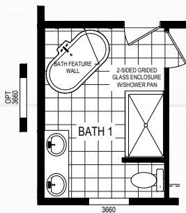
OPTIONAL DELUXE BATH
